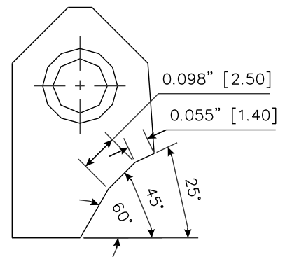
RCA054 Carbide Seat Insert 25-45-60 / 14 -25 RCA-054
