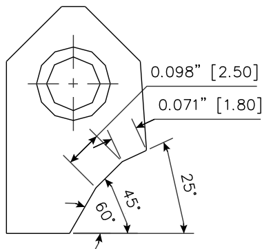
RCA055 Carbide Seat Insert 25-45-60 / 18 -25 RCA-055
