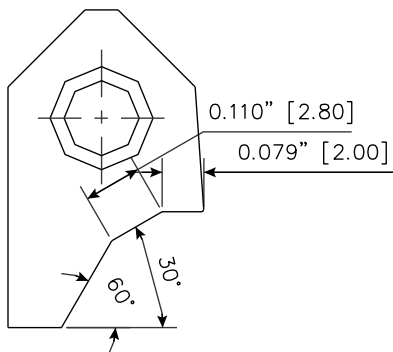
RCA332 Carbide Seat Insert 0-30-60 / 20 -28 RCA-332
