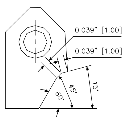
RCA068 Carbide Seat Insert 15-45-60 / 10-10 RCA-068
