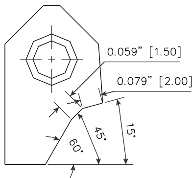
RCA074 Carbide Seat Insert 15-45-60 / 20-15 RCA-074
