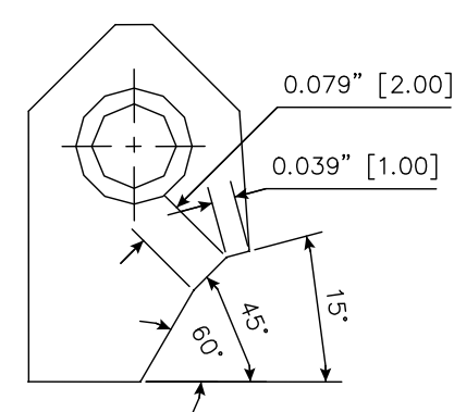
RCA069 Carbide Seat Insert 15-45-60 / 10-20 RCA-069
