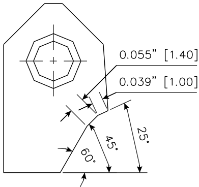
RCA076 Carbide Seat Insert 25-45-60 / 10-14 RCA-076
