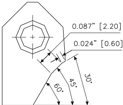
RCA082 Carbide Seat Insert 30-45-60 / 60-22 RCA-082
