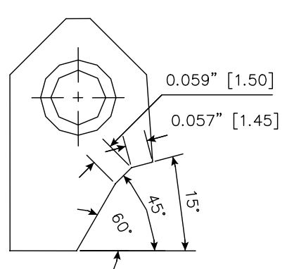
RCA071 Carbide Seat Insert 15-45-60 / 145-15 RCA-071
