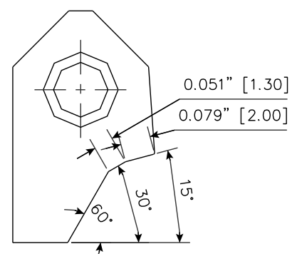
RCA302 Carbide Seat Insert 15-30-60 / 20 -13 RCA-302
