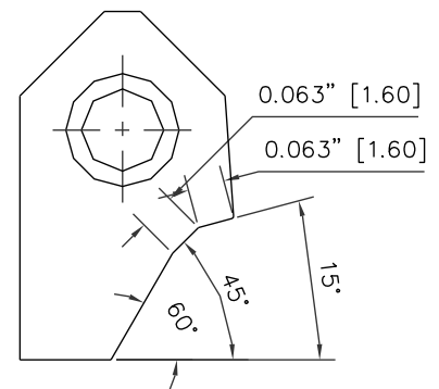
RCA015 Carbide Seat Insert 15-45-60 / 16 -16 RCA-015
