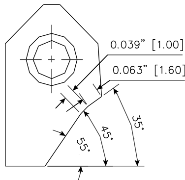
RCA038 Carbide Seat Insert 35-45-55 / 16 -10
