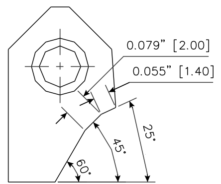
RCA051 Carbide Seat Insert 25-45-60 / 14 -20 RCA-051
