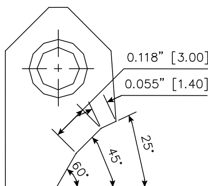
RCA067 Carbide Seat Insert 30-45-60 / 14-30 RCA-067
