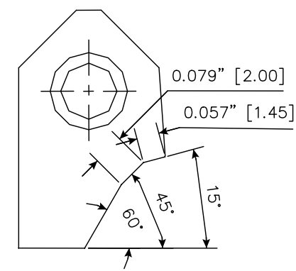
RCA072 Carbide Seat Insert 15-45-60 / 145-20 RCA-072
