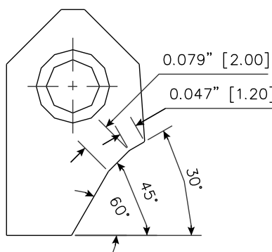
RCA053 Carbide Seat Insert 30-45-60 / 12 -20 RCA-053
