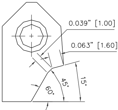
RCA019 Carbide Seat Insert 15-45-60 / 20 -16 RCA-019
