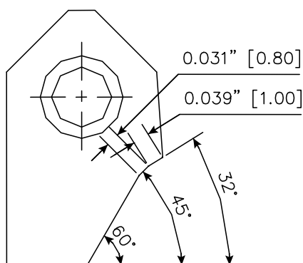
RCA064 Carbide Seat Insert 32-45-60 / 10-80 RCA-064
