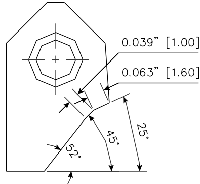
RCA080 Carbide Seat Insert 25-45-52 / 16-10 RCA-080
