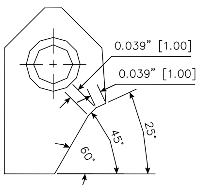
RCA065 Carbide Seat Insert 25-45-60 / 10-10 RCA-065
