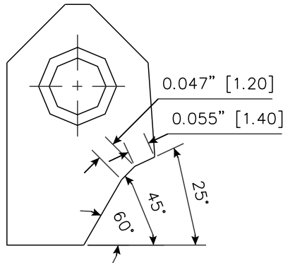
RCA077 Carbide Seat Insert 25-45-60 / 14-12 RCA-077
