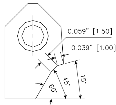
RCA060 Carbide Seat Insert 15-45-60 / 10-15
