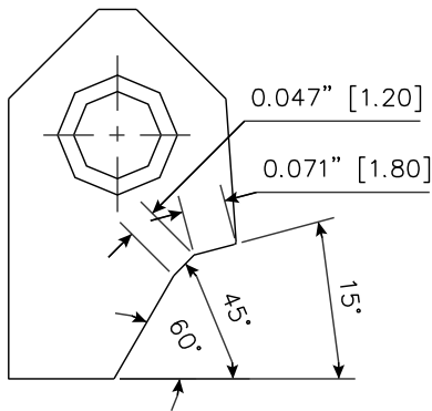
RCA073 Carbide Seat Insert 15-45-60 / 18-12 RCA-073
