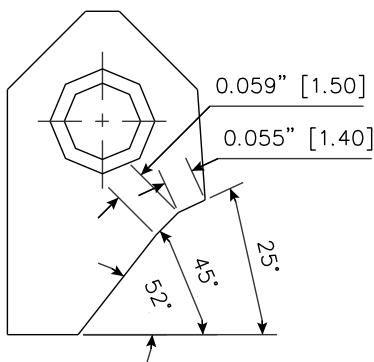
RCA079 Carbide Seat Insert 25-45-52 / 14-15 RCA-079
