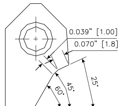
RCA036 Carbide Seat Insert 25-45-60 / 18 -10
