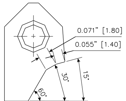
RCA331 Carbide Seat Insert 15-30-60 / 14 -18 RCA-331
