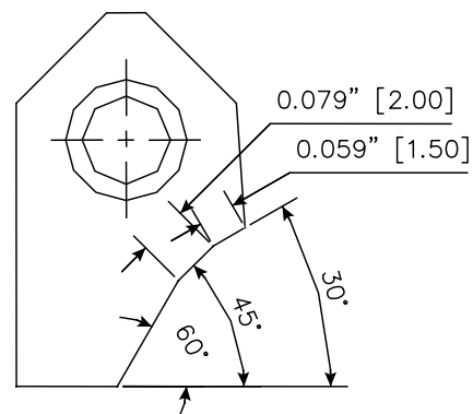
RCA066 Carbide Seat Insert 30-45-60 / 15-20 RCA-066
