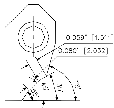
RCA063 Carbide Seat Insert 30-45-55 / 203-151
