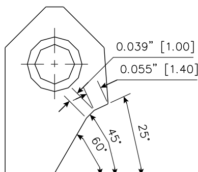
RCA035 Carbide Seat Insert 25-45-60 / 14 -10
