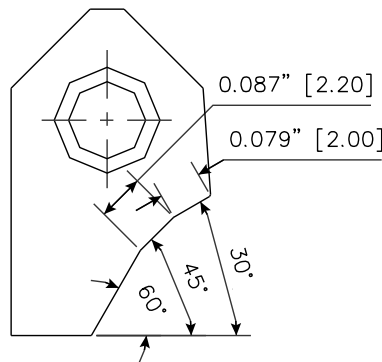
RCA083 Carbide Seat Insert 30-45-60 / 20-22 RCA-083
