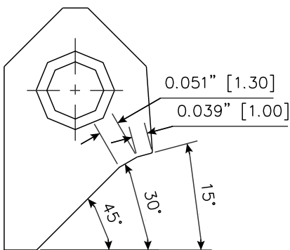
RCA300 Carbide Seat Insert 15-30-45 / 10 -13 RCA-300
