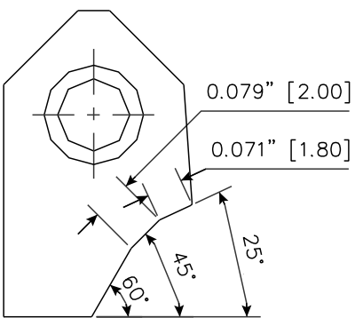
RCA052 Carbide Seat Insert 25-45-60 / 18 -20 RCA-052
