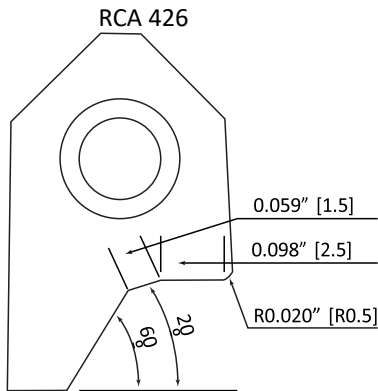
RCA426 Carbide Seat Insert 5-20-60 / 25-15
