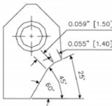
RCA061 Carbide Seat Insert 25-45-60 / 14-15
