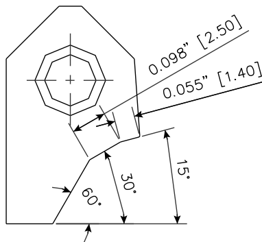
RCA330 Carbide Seat Insert 15-30-60 / 14 -25 RCA-330
